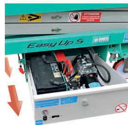
Rationelle Bauteilmontage, wartungsfreundlich.
